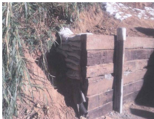
Figura 6.14 Rota 116 – Obra de Contenção – km 66.6
